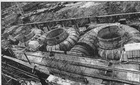
Спиральные камеры седьмой агрегатной секции.
