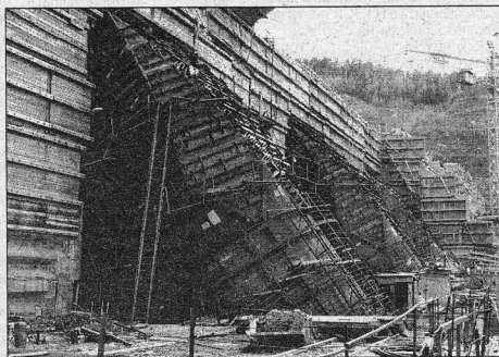
Выкатка звена 9-10 после монтажа.
