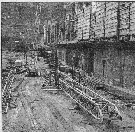
Стрела крана СКР-3500 (68 тонн) подготовлена для монтажа.
