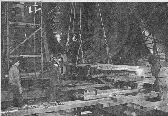
Укрупнительная сборка катучих подмастей для окончательной зачистки звеньев водовода.
