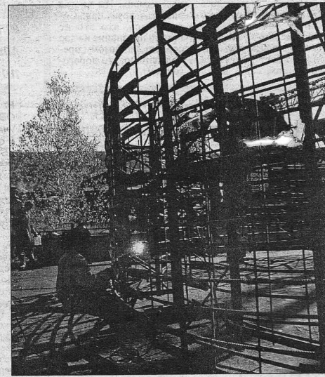
Изготовление армокаркасов.
