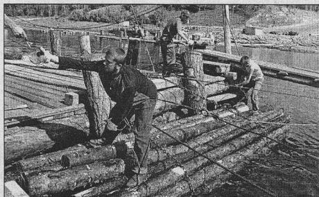
Формировка пучка электролебедкой.
