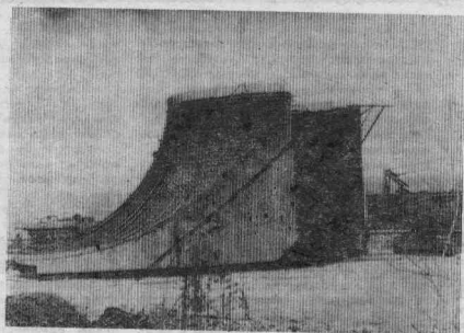
На базе Богучанского участка Братского управления треста «Гидромонтаж» продолжаются работы по изготовлению армокаркаса (на снимке) «торовой части» для первой агрегатной секции Богучанской ГЭС. Их намечается закончить в мае. Фото В. ЗЫКОВА.
