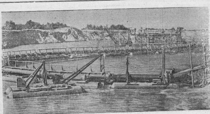
Сталинградгидрострой. Комсомольско-молодежный земснаряд 501 производит выемку грунта и намыл дамбы на трассе нижнего подходного канала к плесу со стороны Волги.
